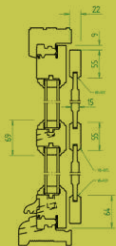
COUPE VERTICALE
